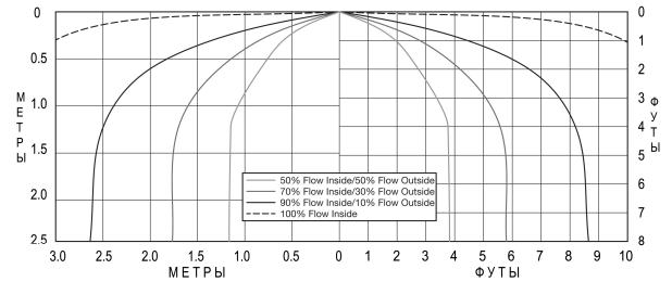
Рис. 7 Карта орошения оросителей TY315/TY313
