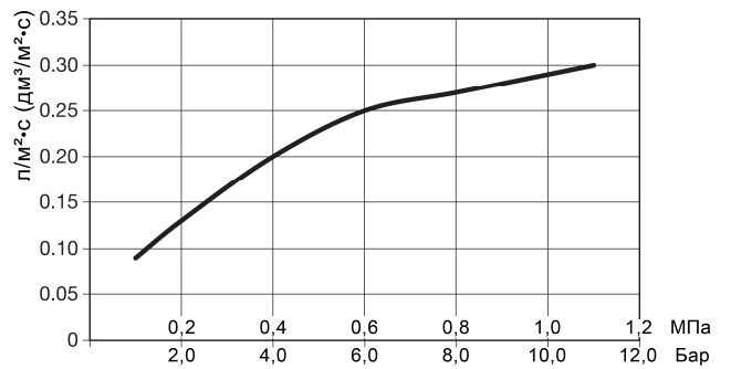
Рис. 9 График зависимости интенсивности орошения оросителей TY315/TY313 от давления (ГОСТ Р 51043-2002)
