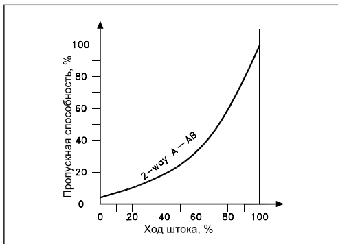
Логарифмическая характеристика для проходных клапанов
